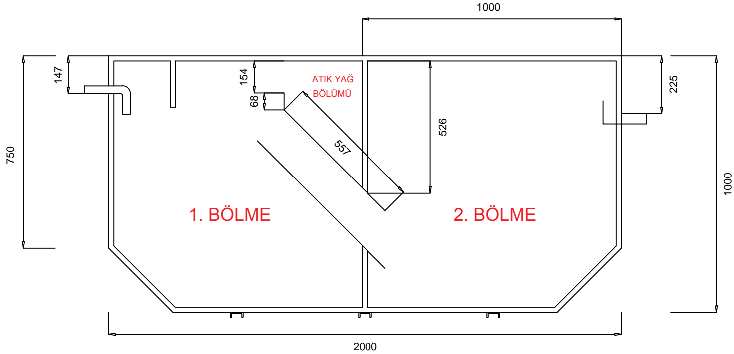
A-A KESİTİ
